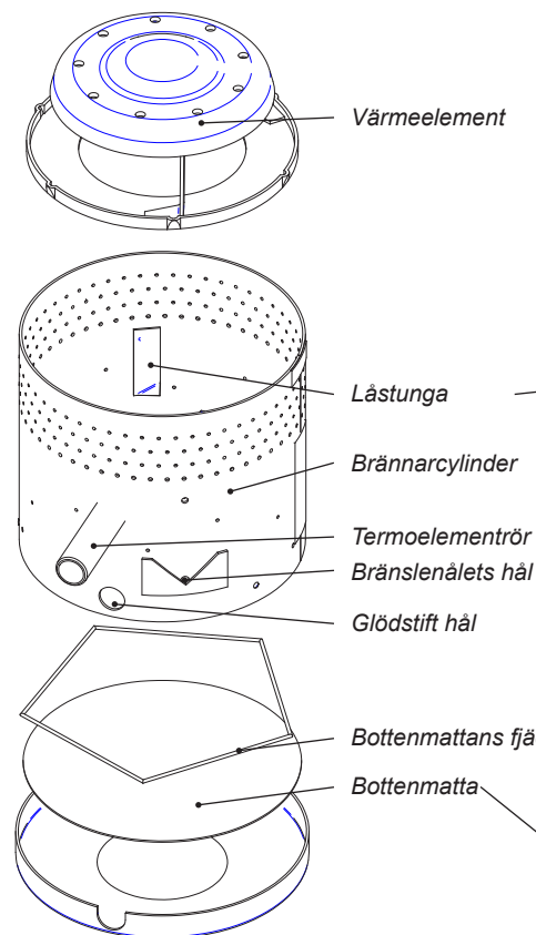
Bild 5. Brännarens komponenter
