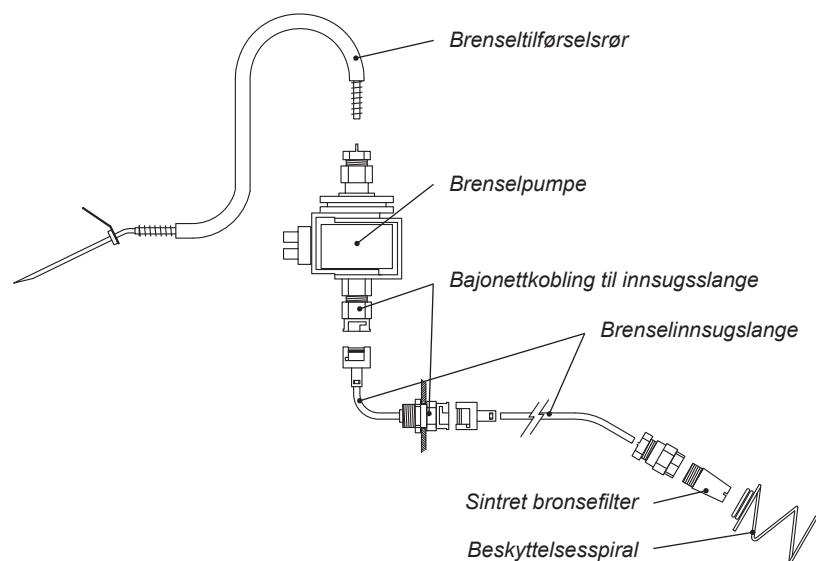
Brenselsystemets bestanddeler
