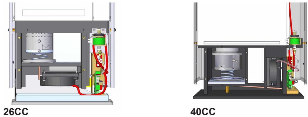
Brännarkammaren öppnad
