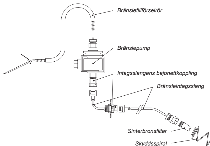
Bränslesystemets komponenter
