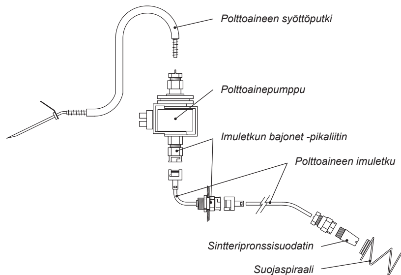
Polttoainejärjestelmän osat
