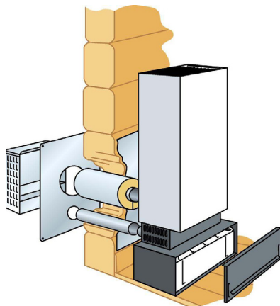
Väggenomföring
