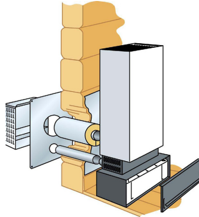
Seinälämpivienti
