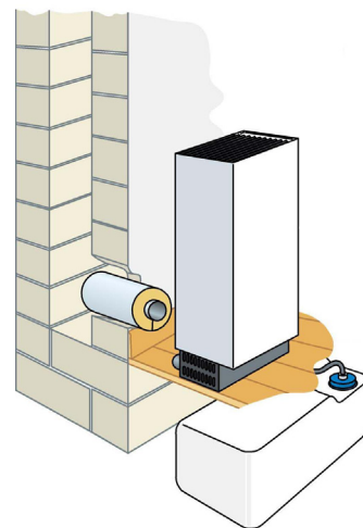
Installering av rökgaskanal.
