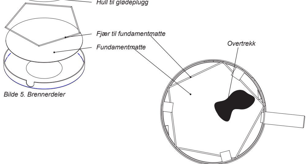
Bilde 7. Brennersylinder
