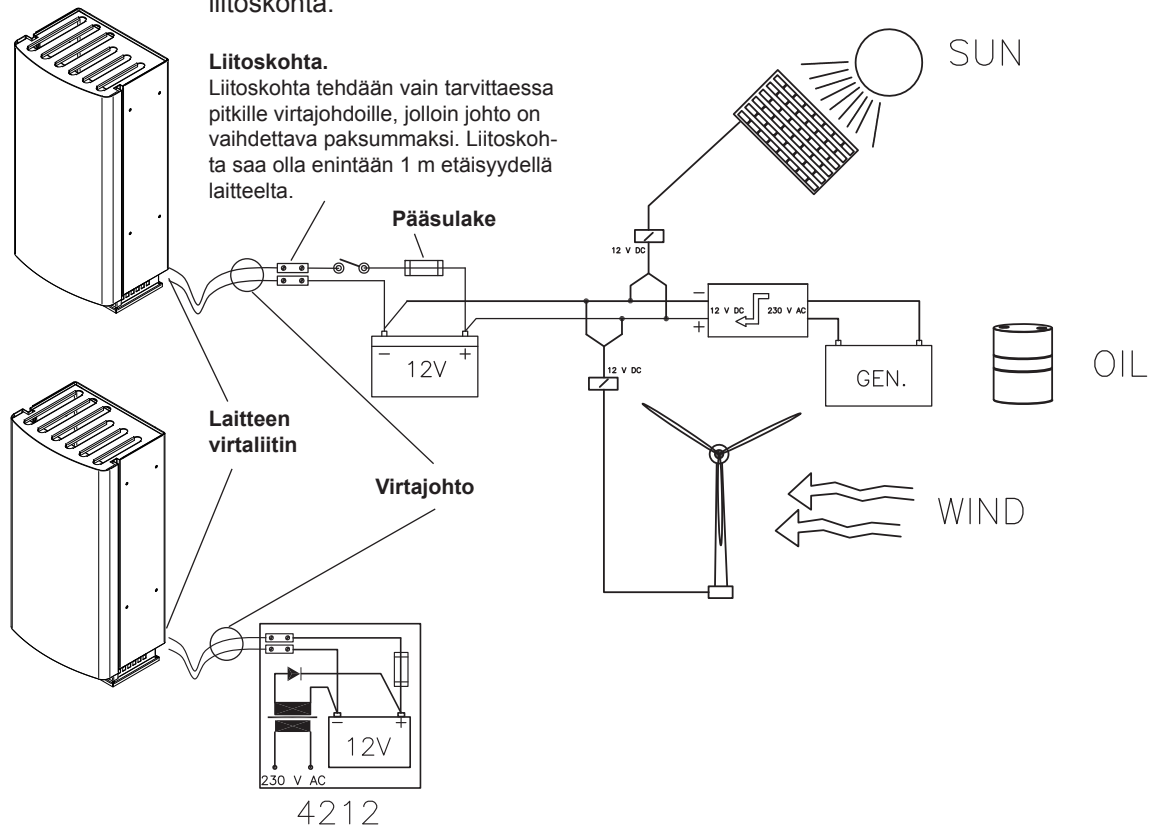
Sähköjärjestelmän periaatekuva.
