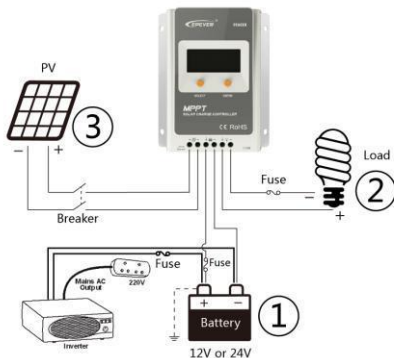
Kuva 2-1 Asennus
